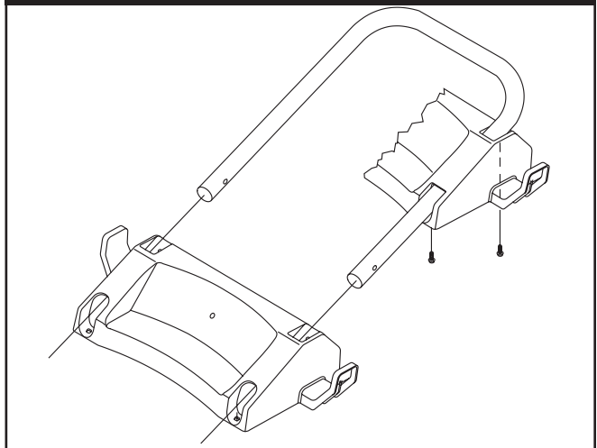
Figura 23 - Conecte Bandeja Accesorias
