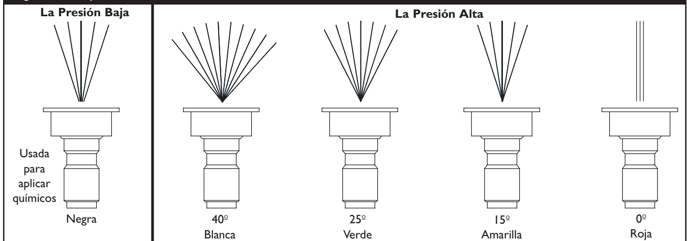
Figura 40 - Boquillas
