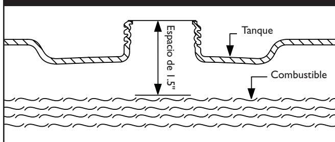
Figura 30 — Espacio Típico para la Expansión del Combustible
