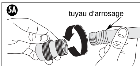
Figure 6 - Raccorder l'autre extrémité de l'adaptateur ( M1 ) à l'arrivée d'eau (« INLET ») ( B ) du nettoyeur, tel qu'illustré. La température de l'eau d'arrivée ne doit PAS dépasser 50 °C (122 °F) et la pression du système d'approvisionnement en eau ne doit PAS être supérieure à 145 lb/po2 (10 bar).
