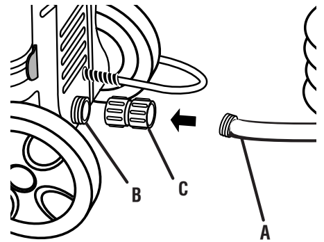
A - Garden hose (tuyau d'arrosage, manguera de jardín) B - Water intake (rise d'eau, entrada de agua) C - Garden hose coupler (raccord de tuyau d'arrosage, acoplador de manguera de jardín)
