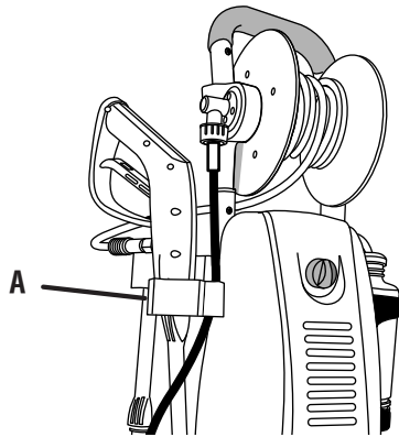
A - Trigger handle and wand storage bracket (poignée à gâchette et support de rangement de la lance, soporte de almacenamiento para el mango del gatillo y el tubo)
