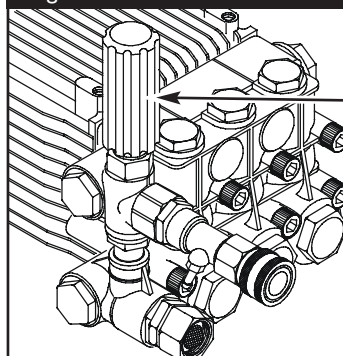
Figura 19 - Perilla Para el Control de la Presión
