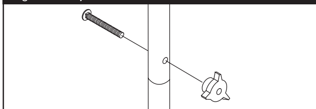
Figura 27 - Sujetar el Manubrio
