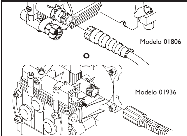
Figura 30 — Conectar la Manguera de Alta Presión a la Toma de Agua
