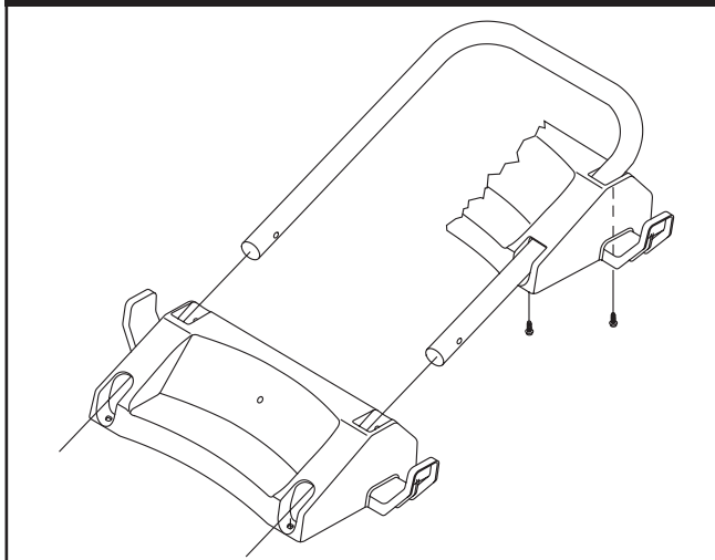
Figura 20 - Conecte Bandeja Accesorio
