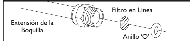
Figura 35 - Limpieza del Filtro
