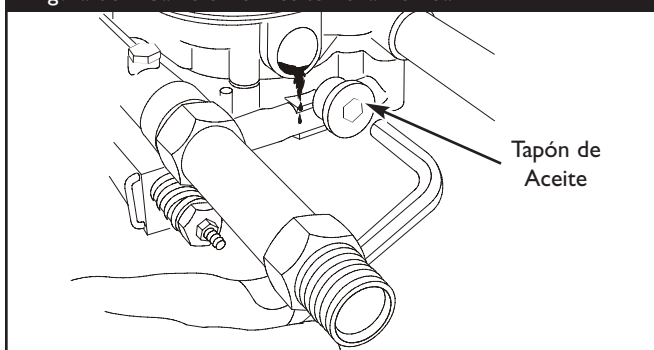
Figura 38 - Cambio del Aceite de la Bomba
