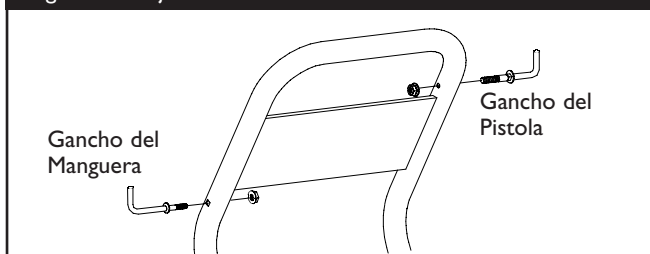
Figura 28 - Fijar el "L" Perno a la Manubrio
