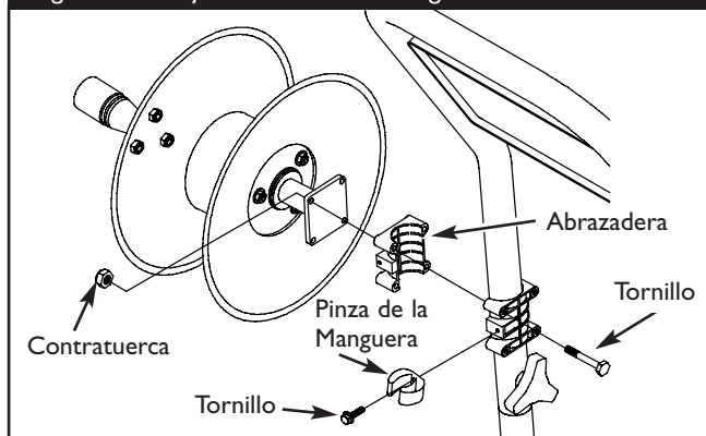
Figura 26 — Fijar el Carretel de Manguera al Asa
