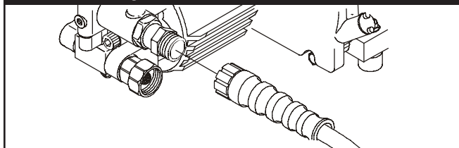
Figura 28 - Conectar la Manguera de Alta Presión a la Toma de Agua
