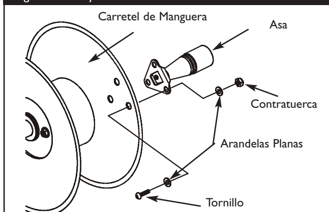
Figura 25 — Fijar Asa al Carretel
