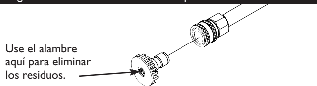
Figura 37 - Mantenimiento de la Boquilla
