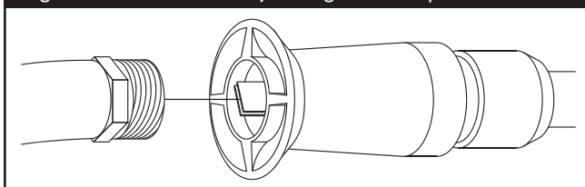
Figura 74 - Suministrar Flujo de Agua a la Boquilla
