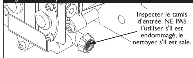
Figure 27 — Inspecter le tamis d'entrée
