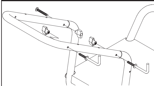
Figure 23 — Fixer les boulons à la poignée
