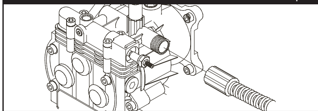
Abb. 46 - Anschließen des Hochdruckschlauchs an der Pumpe
