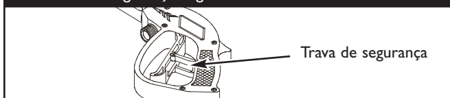
Figura 72 — Pistola de Pulverização com a Trava de Segurança Engatada
