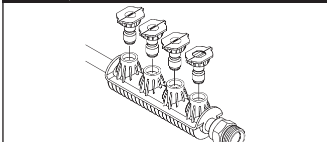
Abb. 51 - Sprühdüsen in Halter einsetzen
