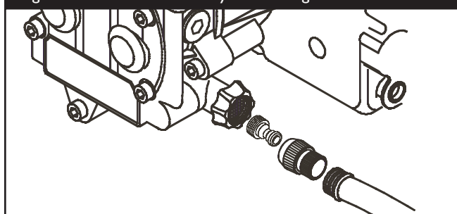
Figure 28 — Connecter le tuyau d'arrosage d'admission d'eau
