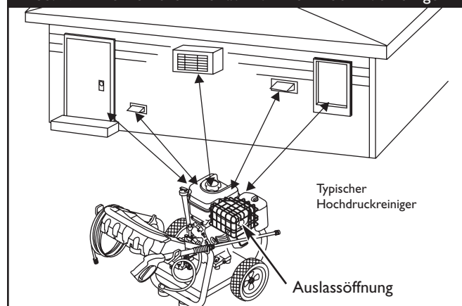
Abb. 49 - Erforderlicher Freiraum um den Hochdruckreiniger
