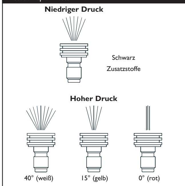
Abb. 56 - Sprühmuster
