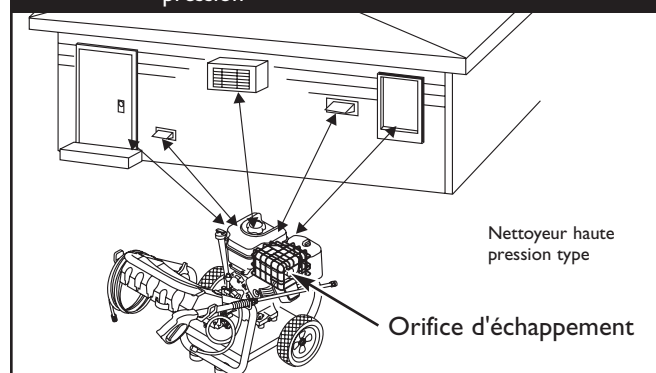
Figure 29 — Débattement autour du nettoyeur haute pression
