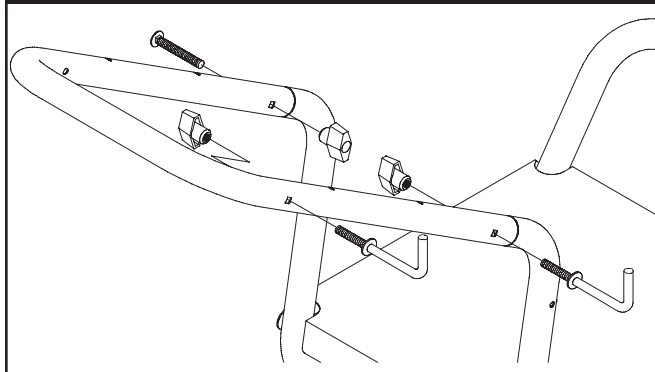
Figura 63 — Fixação dos Parafusos no Puxador
