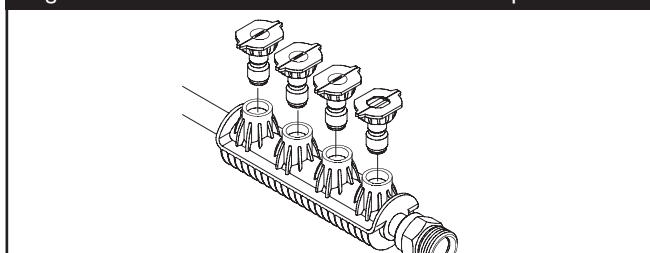
Figura 91 - Instale las Puntas de Rociado en el Soporte
