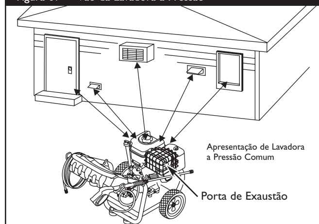
Figura 69 — Vão da Lavadora a Pressão
