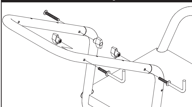
Abb. 43 - Schrauben am Griff befestigen
