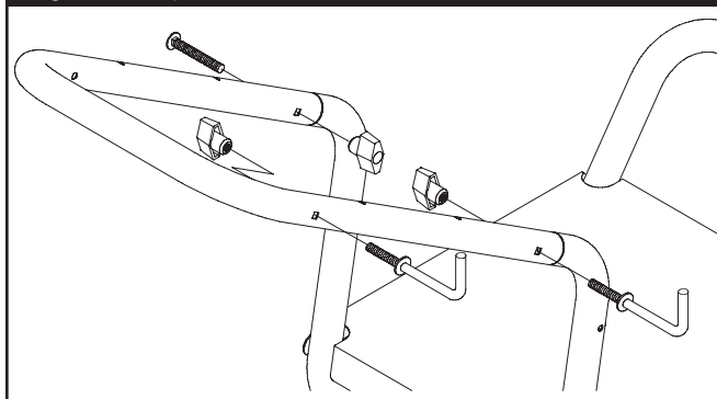
Figura 83 - Fijar el Pernos a la Manubrio
