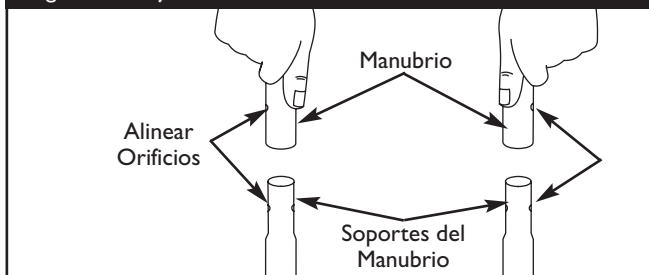
Figura 82 - Fijar el Manubrio a la Base
