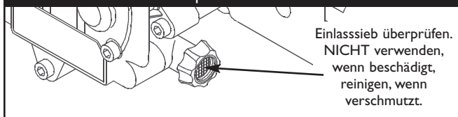
Abb. 47 - Einlasssieb überprüfen
