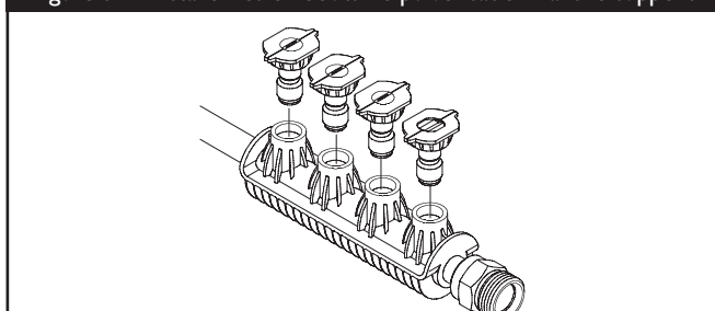
Figure 31 - Installer les embouts de pulvérisation dans le support
