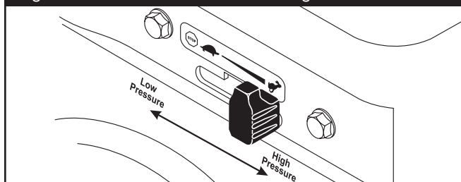
Figura 93 - Palanca de Control de Estrangule
