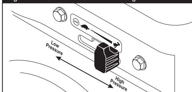
Figura 73 - Alavanca de Controle de Estrangule
