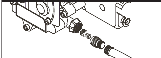
Figura 88 — Conectar la Manguera del Jardín a la Entrada de Agua
