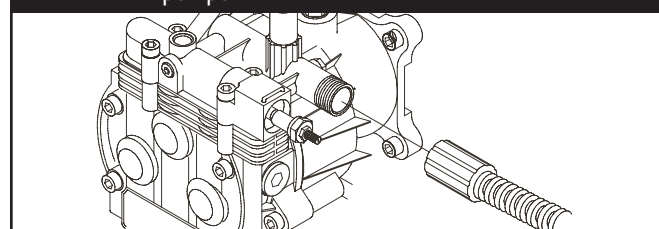
Figure 26 — Connecter l'autre tuyau de pression pour pomper
