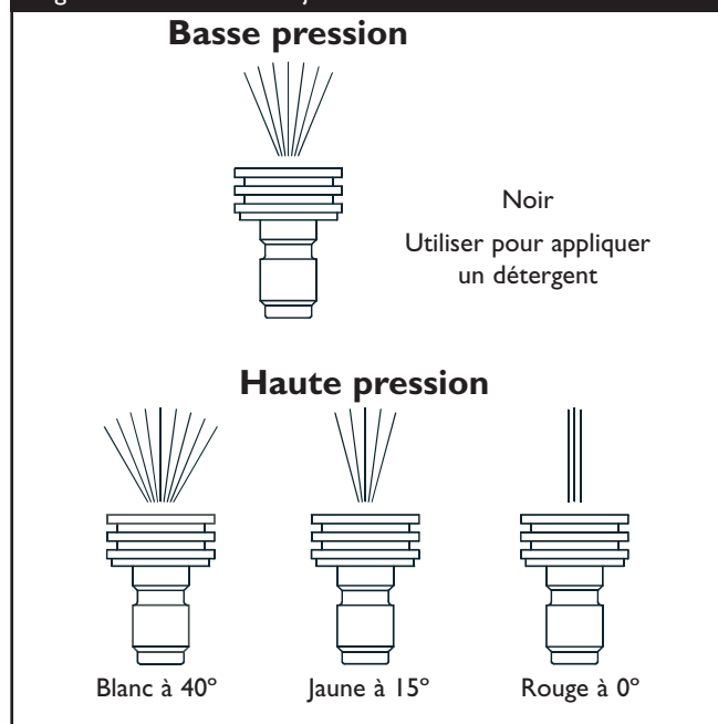
Figure 36 — Formes de jet selon l'embout choisi
