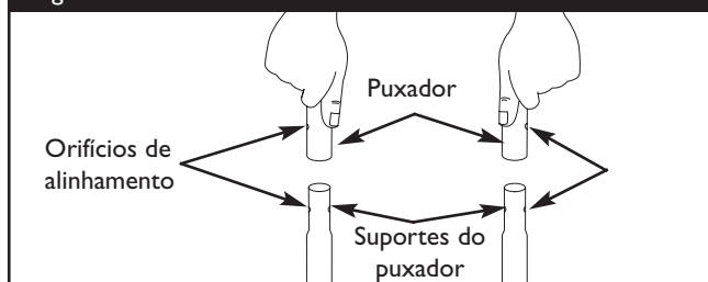
Figura 62 — Conecte o Puxador à Base
