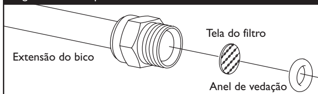
Figura 78 — Limpe o Filtro de Linha
