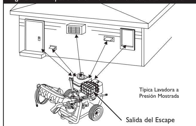
Figura 89 — Espacio Libre Alrededor del Lavadora a Presión
