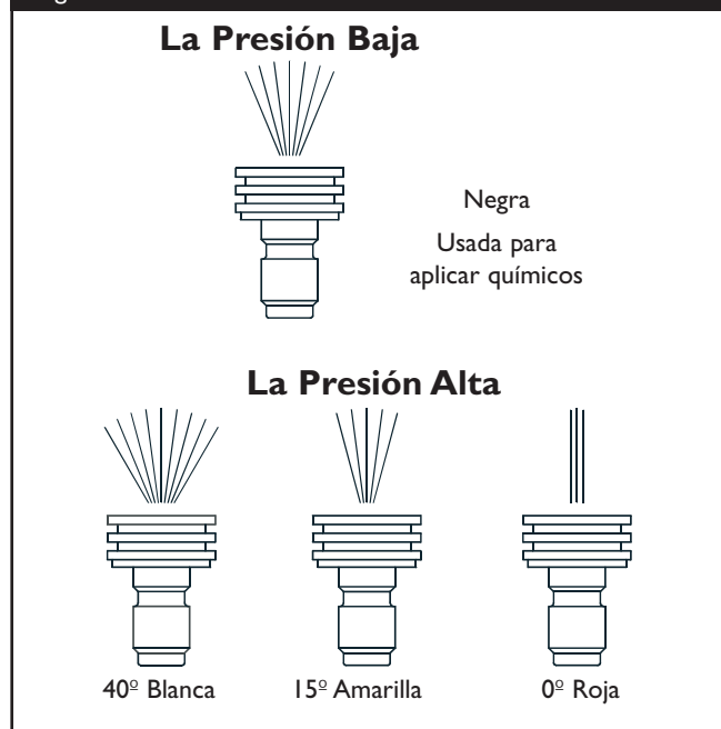
Figura 96 — Rocío los Modelos del Rocío de Punta
