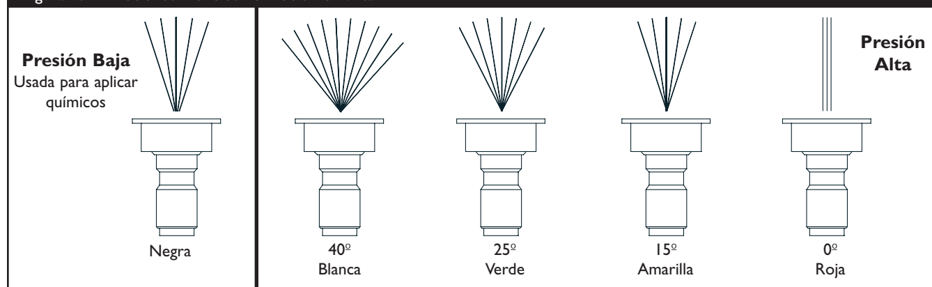
Figura 73 — Rocíe los Modelos del Rocío de Punta
