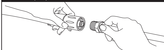
Abb. 40 - Anschließen der Düsenverlängerung an der Spritzpistole
