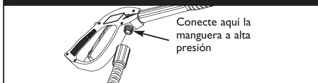
Figura 25 — Conecte la Manguera a alta Presión a la Pistola Rociadora
