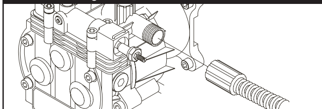
Figura 30 - Conectar la Manguera de Alta Presión a la Toma de Agua
