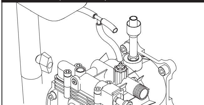
Figura 28 — Conecte la Manguera para Productos Químicos al Acoplamiento de Inyección de Productos Químicos
