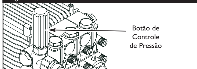
Figura 75 — Botão de Controle de Pressão
