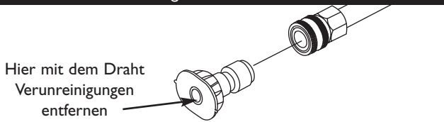
Abb. 59 - Düsenwartung
