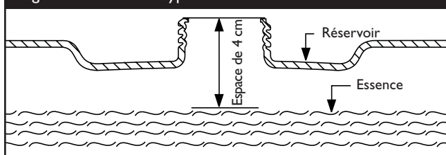
Figure 26 — Volume-type de dilatation du carburant
