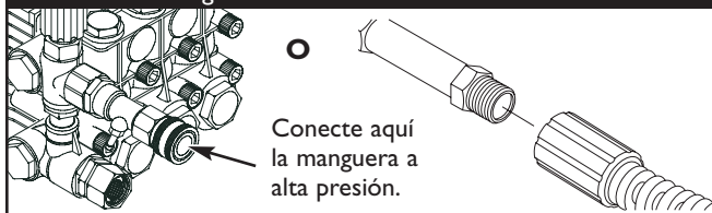
Figura 88 - Conectar la Manguera de Alta Presión a la Toma de Agua
