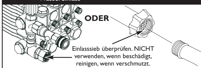
Abb. 49 - Anschließen des Gartenschlauchs an den Wassereinlass
