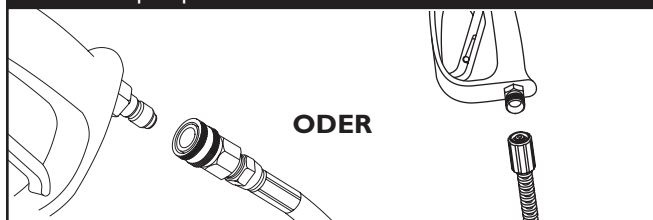
Abb. 47 - Anschließen des Hochdruckschlauchs an der Spritzpistole
