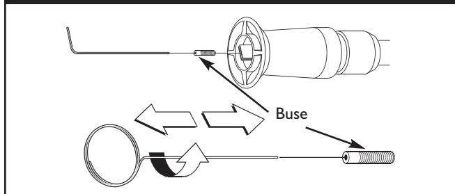
Figura 77 — Remova e Limpe o Bico
