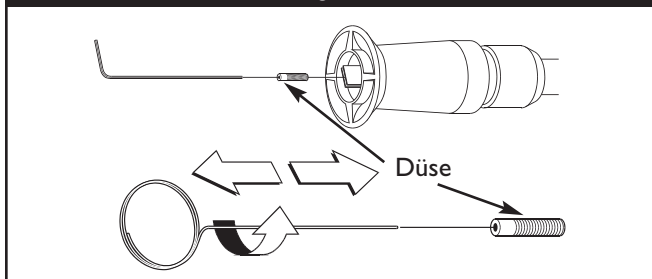
Abb. 57 - Ausbauen und Reinigen der Düse
