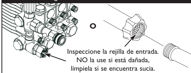
Figura 89 - Conecte la Manguera para el Jardín, a la Entrada de Agua
