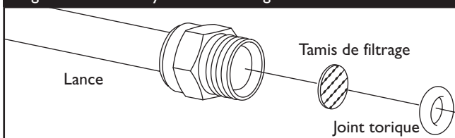
Figure 36 — Nettoyer le filtre en ligne
