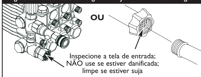
Figura 69 — Conecte a Mangueira de Jardim à Entrada de Água
