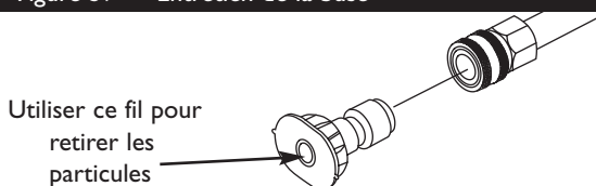
Figure 39 — Entretien de la buse
