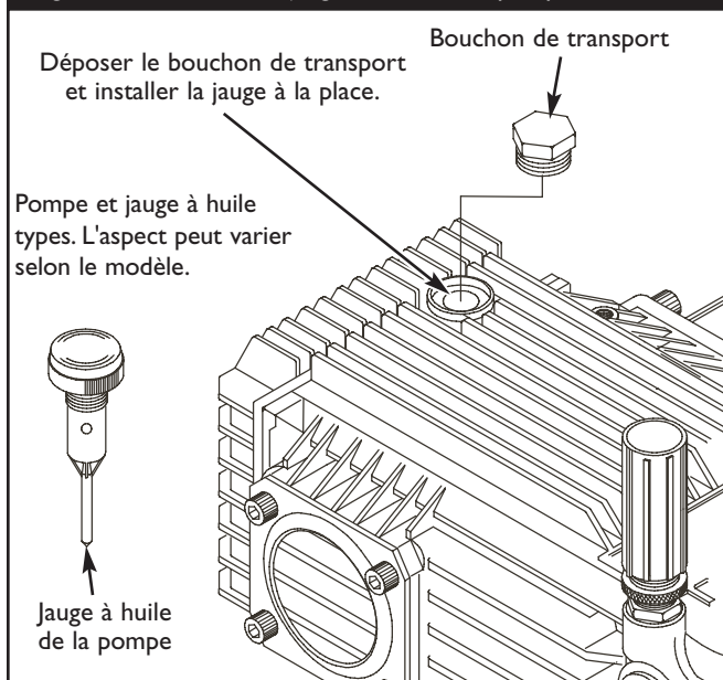
Figure 25 — Monter la jauge à huile sur la pompe
