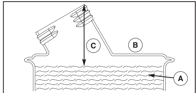
Figura 3 — Expansión del combustible
