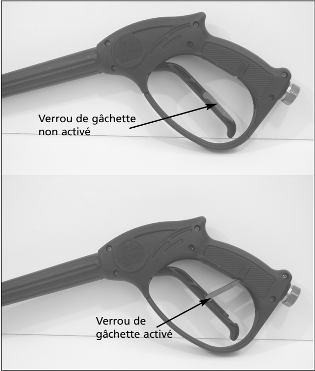
Figure 11 - Verrou de gâchette
