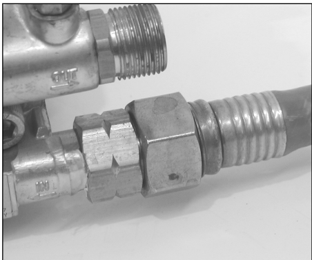
Figure 6 - Fixez le tuyau d'arrosage
