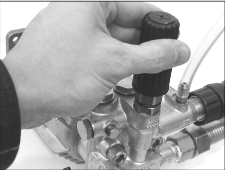
Figura 13 – Ajuste de la presión de la bomba axial
