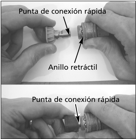
Figure 15 - Instalación de la punta de conexión rápida
