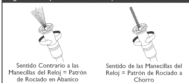
Figura 28 — Ajustar el Patrón de Aspersión
