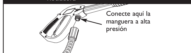
Figura 20 — Conecte la Manguera a alta Presión a la Pistola Rociadora
