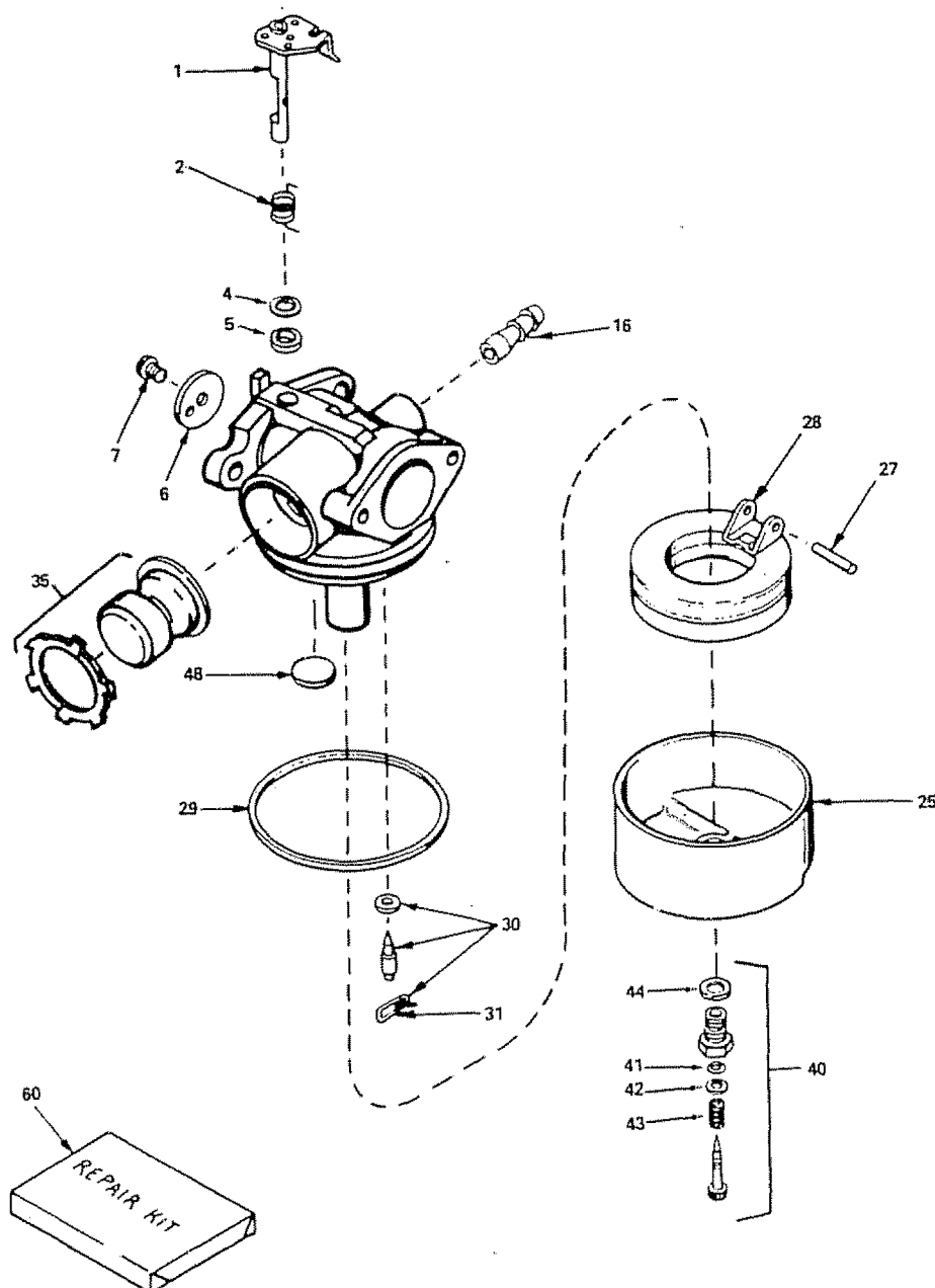
Carburador No. 632589
