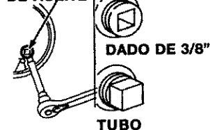
TAPÓN DE LLENADO DE ACEITE
