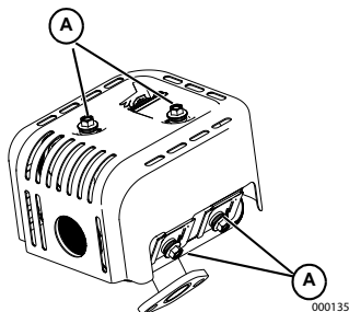
Figura 4-9. Fijaciones del protector de calor
