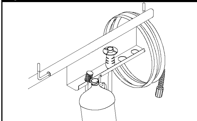
Figura 37 - Charola de Accesorios sobre el Charola Accesoría
