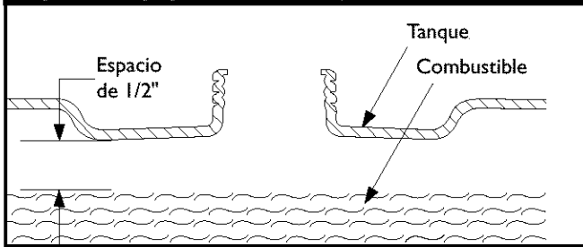
Figura 30 - Agregar Gasolina al Tanque de Combustible
