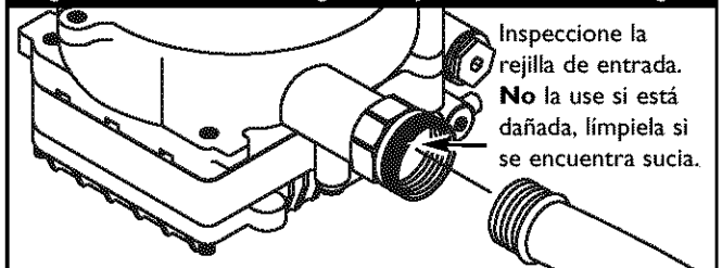
Figura 34 - Conectar la Manguera del Jardín a la Entrada de Agua
