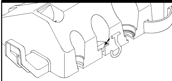
Figura 27 - Colocar el Gancho "J" Hook sobre el Charola de Accesorio
