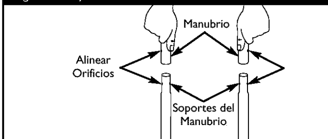
Figura 25 - Fijar el Manubrio a la Base
