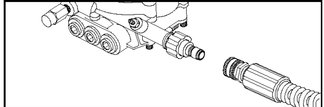
Figura 32 - Conectar la Manguera de Alta Presión a la Toma de Agua
