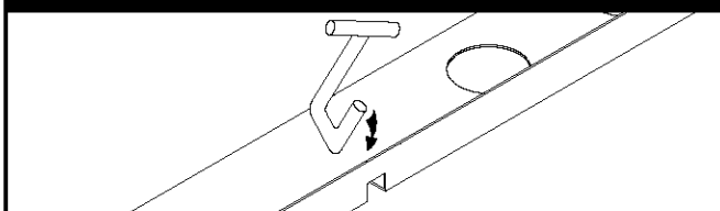
Figura 25 - Colocar el gancho "J" Hook sobre el Charola Accesorio
