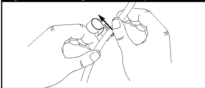
Figura 26 - Deslice Manga Química en el Clip de Metal
