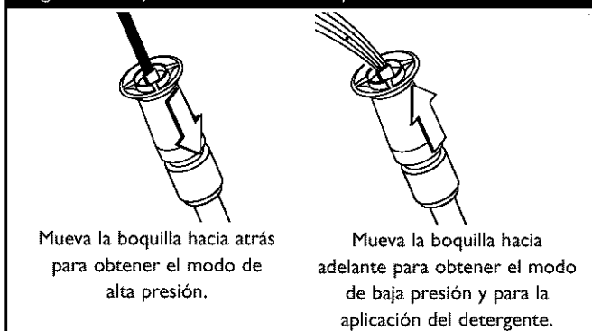
Figura 38 - Ajustar la Presión de Aspersión
