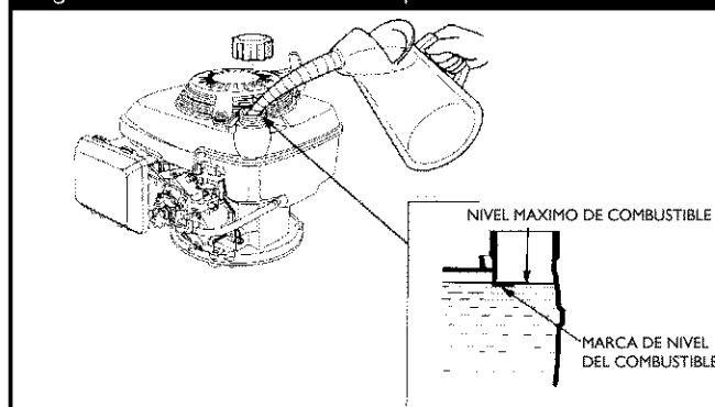
Figura 28 - Añada Gasolina al Tanque de Combustible
