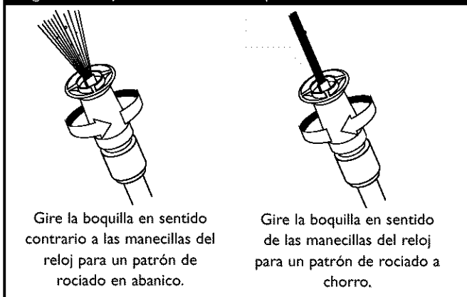
Figura 40 - Ajustar el Patrón de Aspersión
