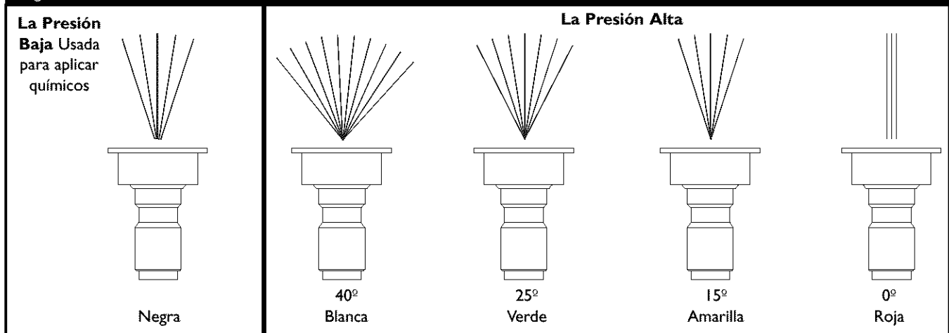
Figura 16 - Puntas de Rocío
