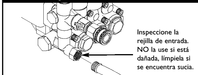
Figura 13 - Conecte la Manguera para el Jardín, a la Entrada de Agua
