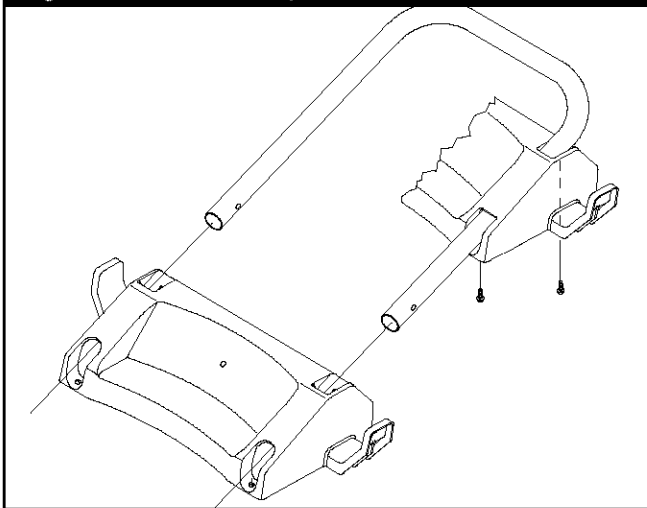
Figura 22 - Conecte Bandeja Accesorio
