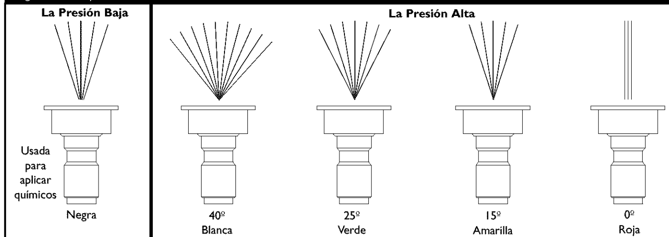
Figura 38 - Boquillas
