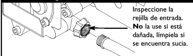
Figura 32 - Conecte la Manguera para el Jardín, a la Entrada de Agua
