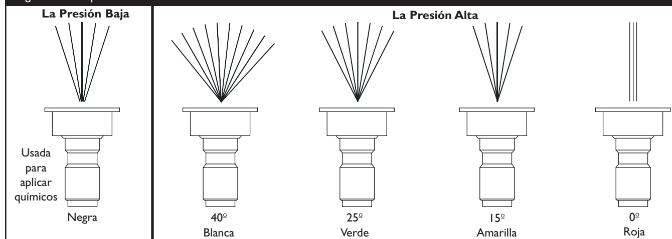
Figura 39 - Boquillas
