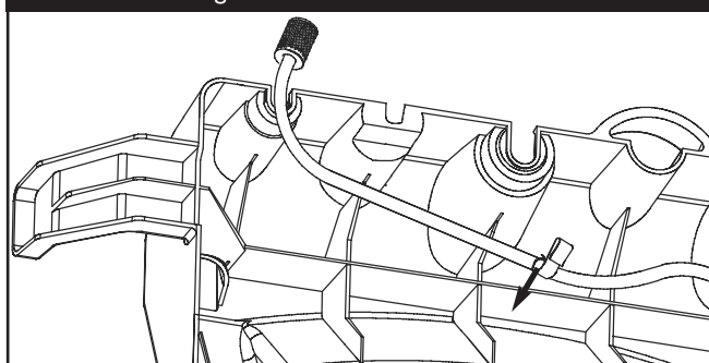
Figure 29 — Deslice Clip de Metal en la Bandeja Accesorio Flange
