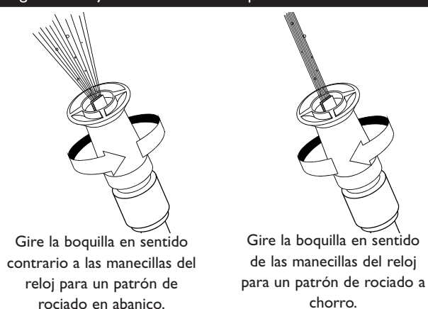
Figura 28 - Ajustar el Patrón de Aspersión
