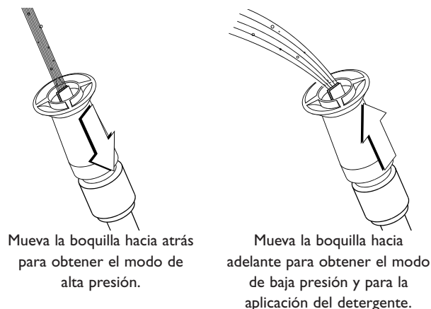
Figura 26 - Ajustar la Presión de Aspersión
