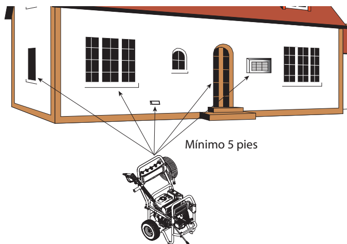
Figura 19 - Espacios libres
