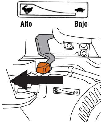
Figura 22 – Control del obturador
