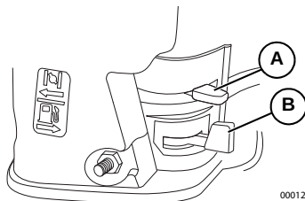
Figure 3-2. Robinet de carburant et levier d'étranglement
