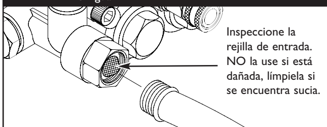
Figura 16 - Conecte la Manguera para el Jardín, a la Entrada de Agua
