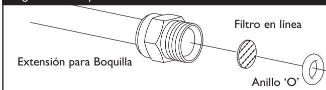
Figura 21 - Limpieza del Filtro
