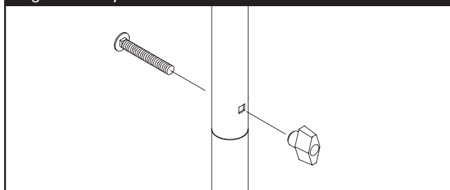
Figura 17 - Sujetar el Manubrio
