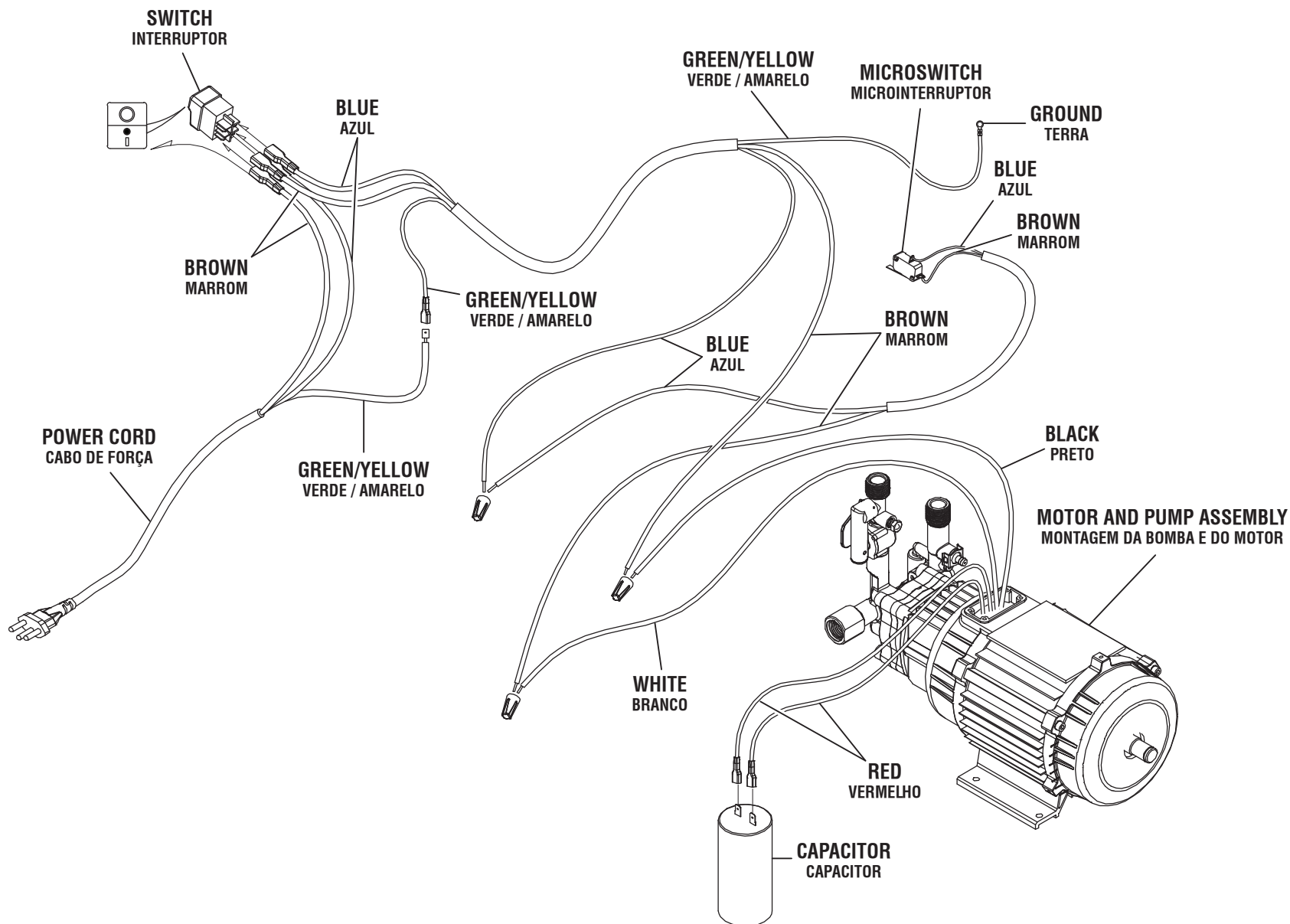
WIRING DIAGRAM DIAGRAMA DE FIAÇÃO
