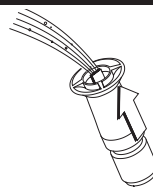
Figura 26 — Ajustar la Presión de Aspersión
