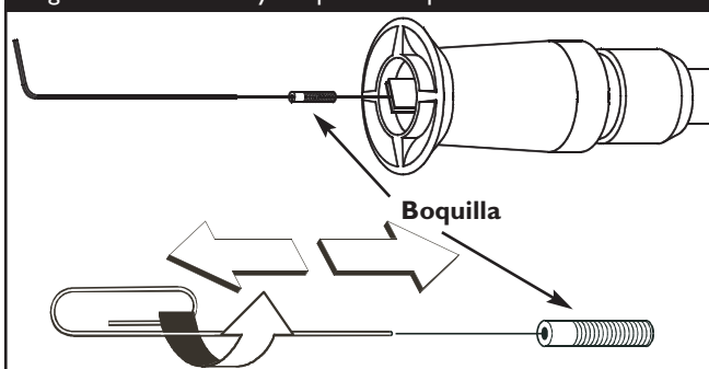
Figura 30 - Remover y Limpiar la Boquilla
