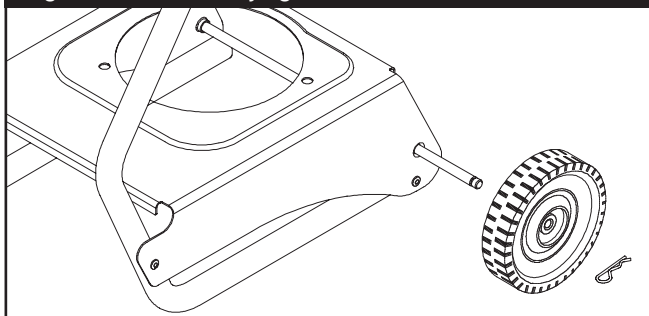
Figura 17 — Instale el Juego de Ruedas
