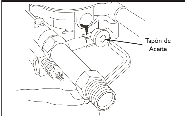
Figura 30 - Cambio del Aceite de la Bomba
