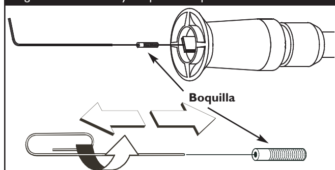
Figura 28 - Remover y Limpiar la Boquilla
