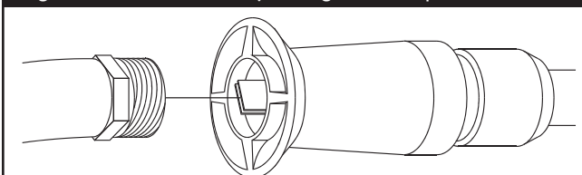
Figura 29 - Suministrar Flujo de Agua a la Boquilla
