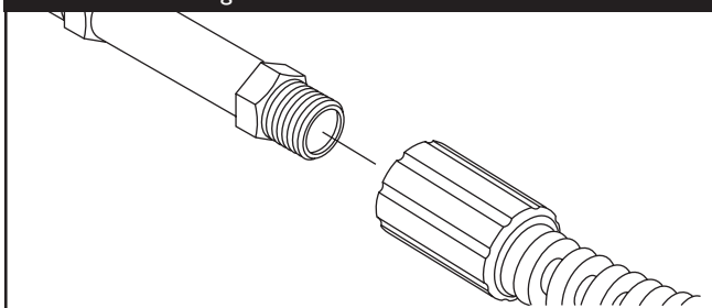
Figura 20 — Conectar la Manguera de Alta Presión a la Toma de Agua
