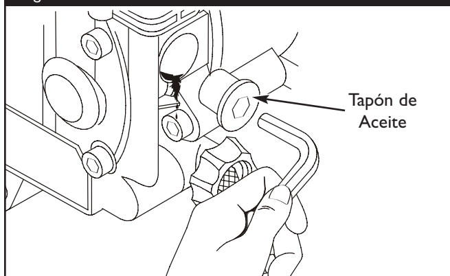
Figura 28 - Cambio del Aceite de la Bomba
