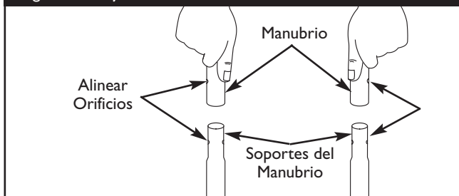
Figura 15 - Fijar el Manubrio a la Base
