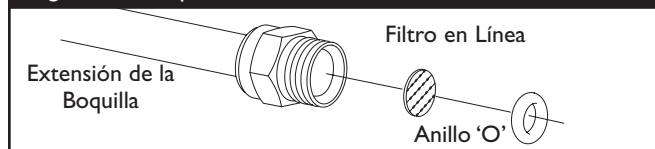
Figura 27 - Limpieza del Filtro
