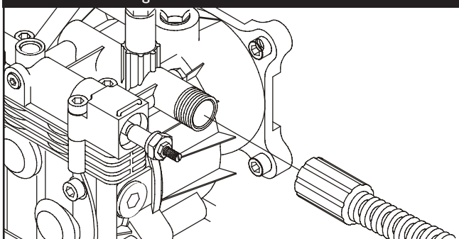
Figura 20 — Conectar la Manguera de Alta Presión a la Toma de Agua
