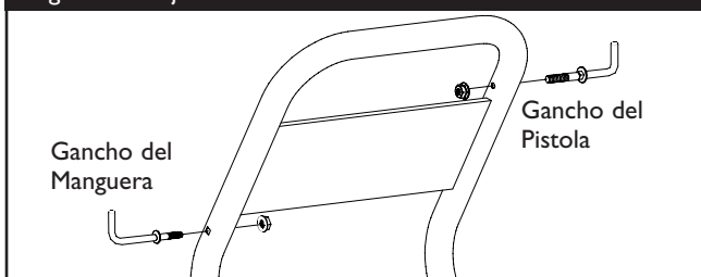
Figura 17 - Fijar el "L" Perno a la Manubrio
