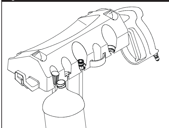
Figura 35 - Charola de Accesorios Sobre el Charola Accesoria
