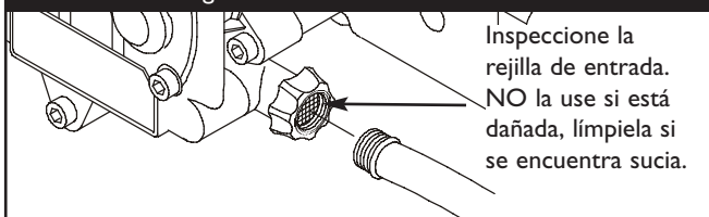
Figura 31 - Conecte la Manguera para el Jardín, a la Entrada de Agua
