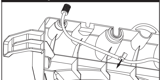
Figure 27 — Deslice Clip de Metal en la Bandeja Accesorio Flange
