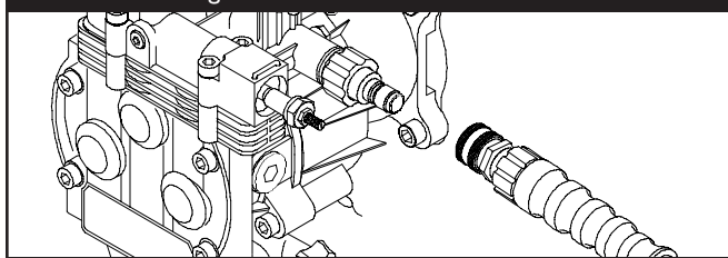
Figura 29 - Conectar la Manguera de Alta Presión a la Toma de Agua
