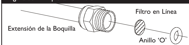
Figura 38 - Limpieza del Filtro
