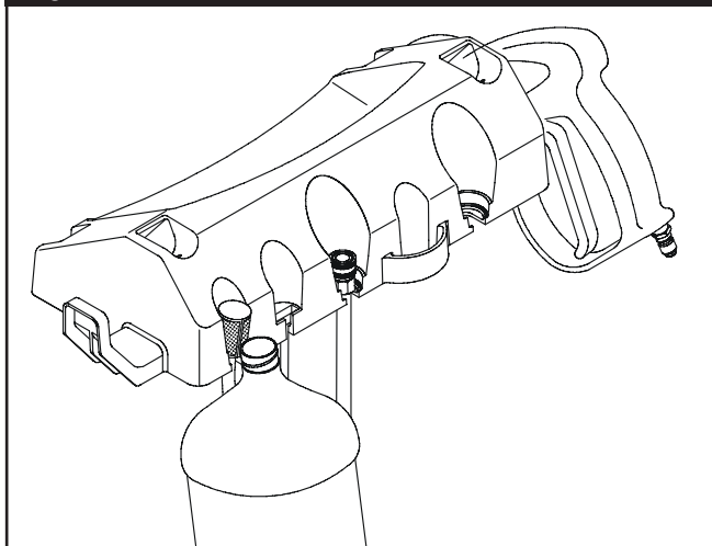
Figura 33 - Charola de Accesorios Sobre el Charola Accesoría
