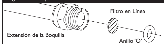
Figura 40 - Limpieza del Filtro
