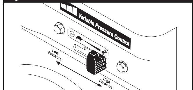
Figura 35 - Control de la Válvula de Admisión
