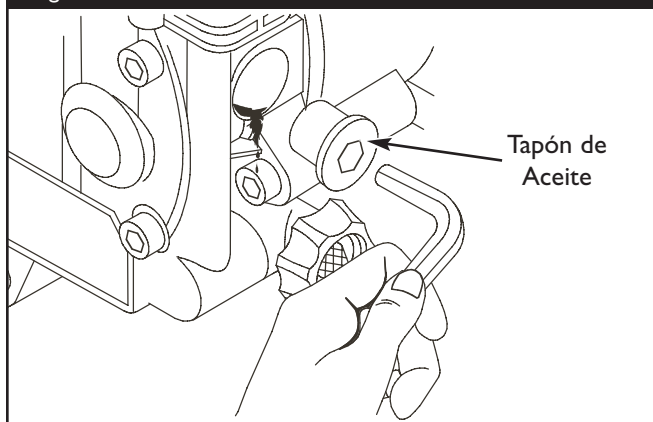
Figura 43 - Cambio del Aceite de la Bomba
