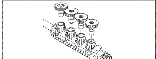
Figura 34 - Instale Puntas de Rocío en el Poseedor
