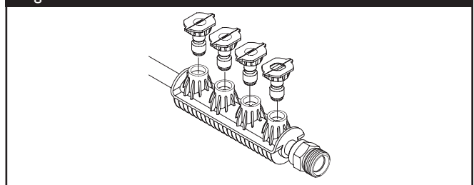
Figura 26 - Instale Puntas de Rocío en el Poseedor
