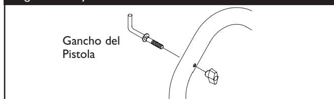
Figura 28 - Fijar el "L" Perno a la Manubrio
