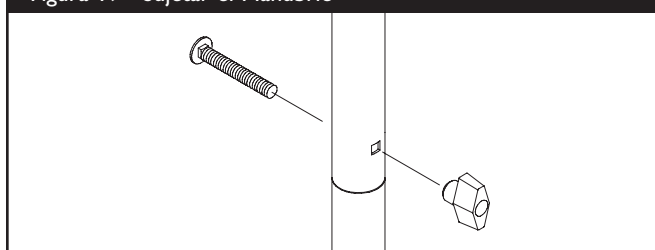
Figura 19 - Sujetar el Manubrio
