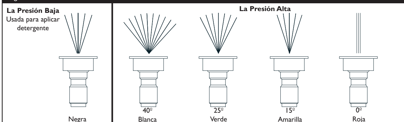
Figura 27 - Punta de Rociado
