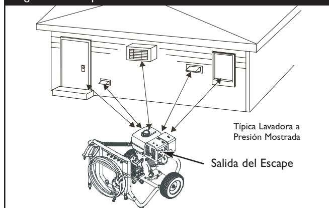
Figura 23 — Espacio Libre Alrededor del Lavadora a Presión
