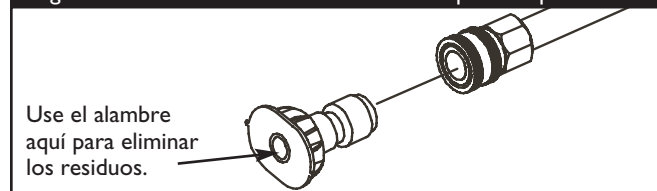
Figura 30 - Mantenimiento de la Extensión para Boquilla
