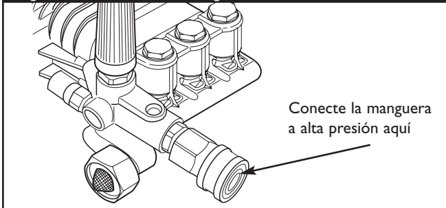
Figura 21 — Conecte la Manguera a Alta Presión, a la Bomba
