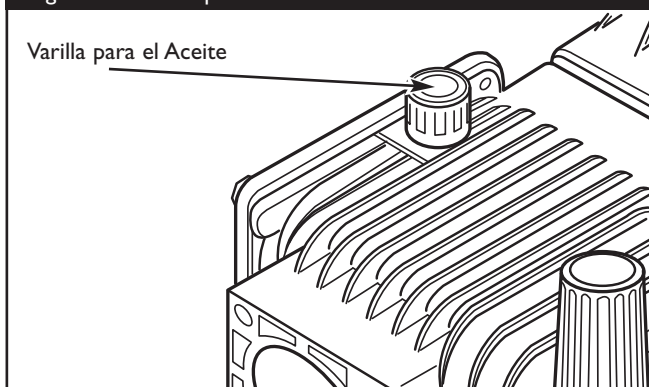
Figura 17 - Varilla para el Aceite en la Bomba
